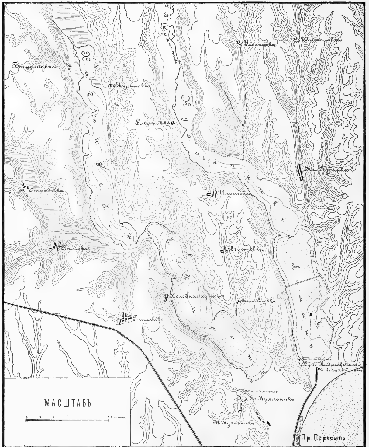
Куйалницкій и Хаджибейскій лиманы. Die Limane: Kujalnik u. Hadshibey. Горизонтали черезъ 10 метровъ, глубины въ метрахъ.
